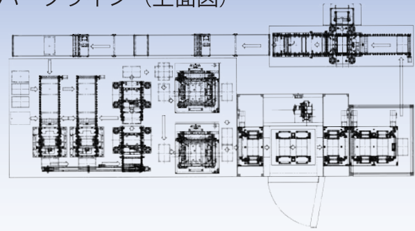
ハーフライン (上面図)
